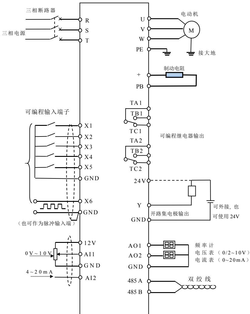
图 2-6 基本运行配线图
