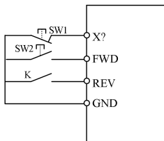
b) 三线控制模式 2 接线图
