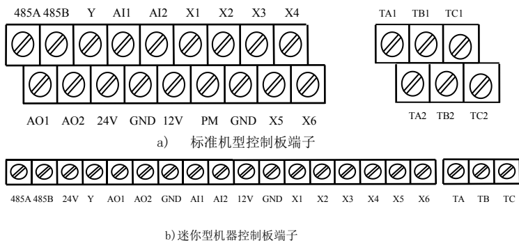
图 2-5 控制回路端子台配线图
