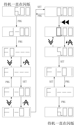
图 3-1 修改功能参数流程图
