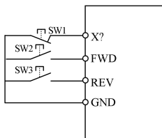
a) 三线控制模式 1 接线图
