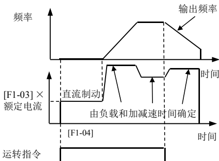
图 1 直流制动方式起动机
